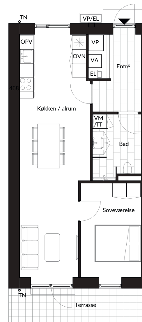
Boligplan - 65 m2
